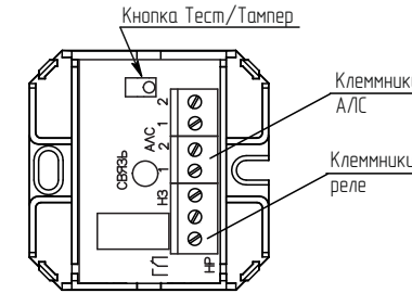
Рисунок 1- Модуль релейный РМ-1 прот. R3
