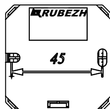
Рисунок 5 – Установочные размеры для PM-1 прот. R3
