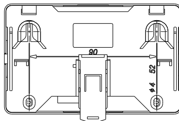
Рисунок 4 – Установочные размеры для PM-1C прот. R3, PM-4 прот. R3
