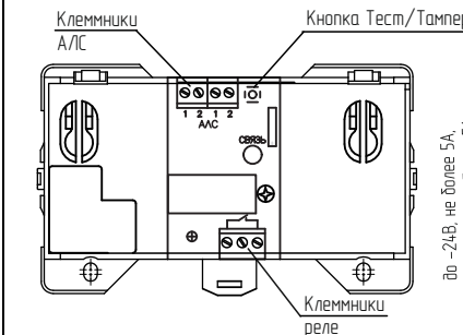
Рисунок 3- Модуль релейный РМ-1C прот. R3
