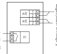
Рисунок 3- Модуль релейный РМ-1C прот. R3
